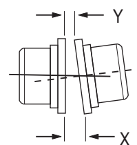
Desalinhamento Angular
