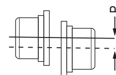
Desalinhamento Paralelo
